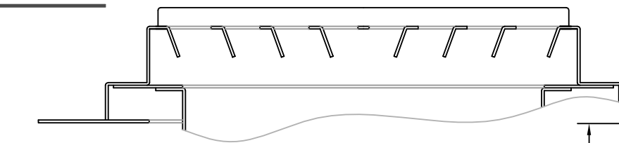
F-F 断面
