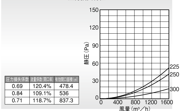
圧力損失特性
