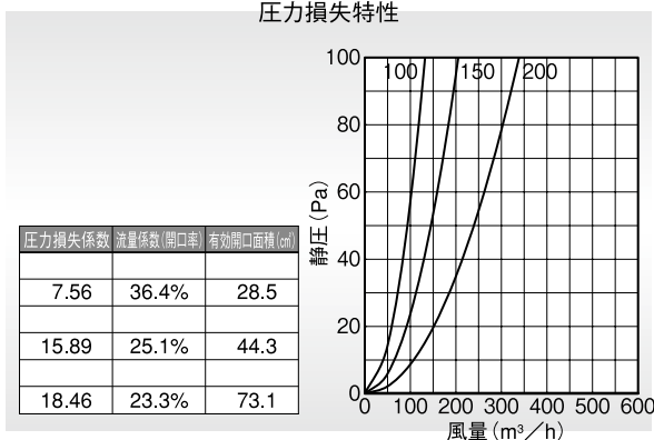
圧力損失特性
