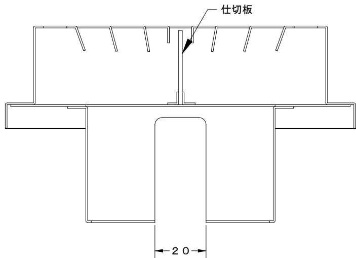
A-A 断面
