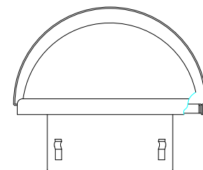
G 矢視図
