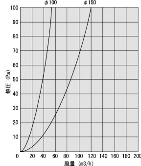
RCND-TBSC 圧力損失特性
