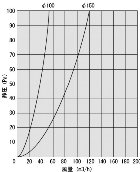
RCN-TBS 圧力損失特性
