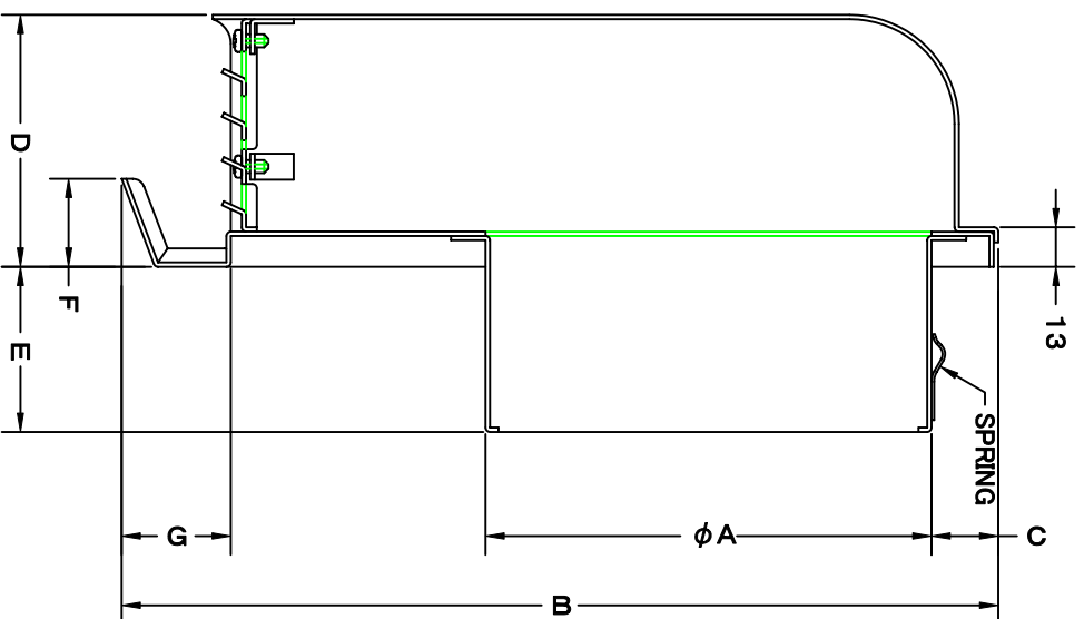
K 矢视图
