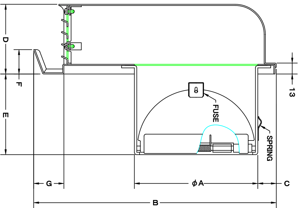
K 矢视图
