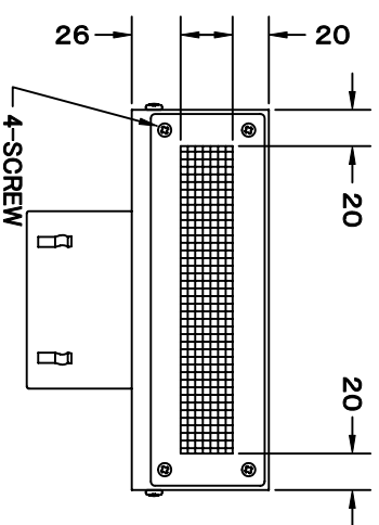
F 矢视图 (1/2)
