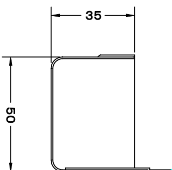
水溜部詳細
