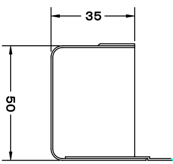
水溜部詳細
