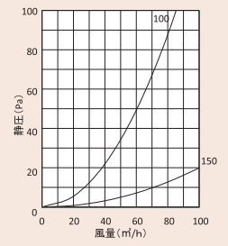
圧力損失特性
